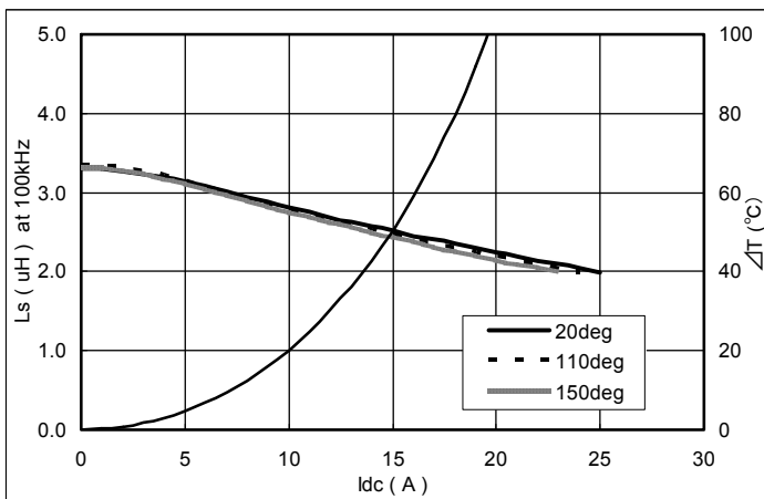
CDMC10D50T150NP-3R3M
